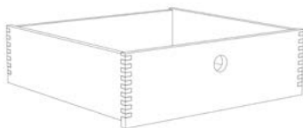
K-Fräsung
